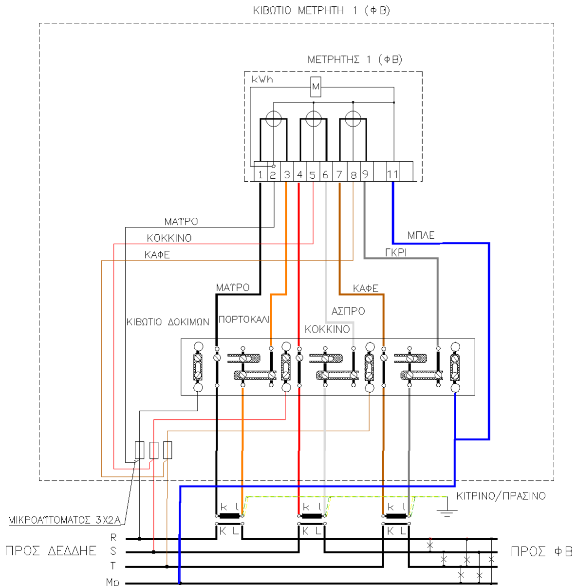
Σχήμα 4: Μονογραμμικό Διάγραμμα Μετρητικής Διάταξης τριφασικού μετρητή ΦΒ ισχύος 55 kWp έως 250 kWp
